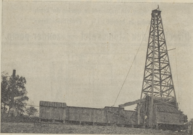
EEN „OILWELL” STANDAARD KABEL-INRICHTING.
